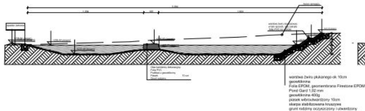
PRZEKRÓJ ST1-ST1
